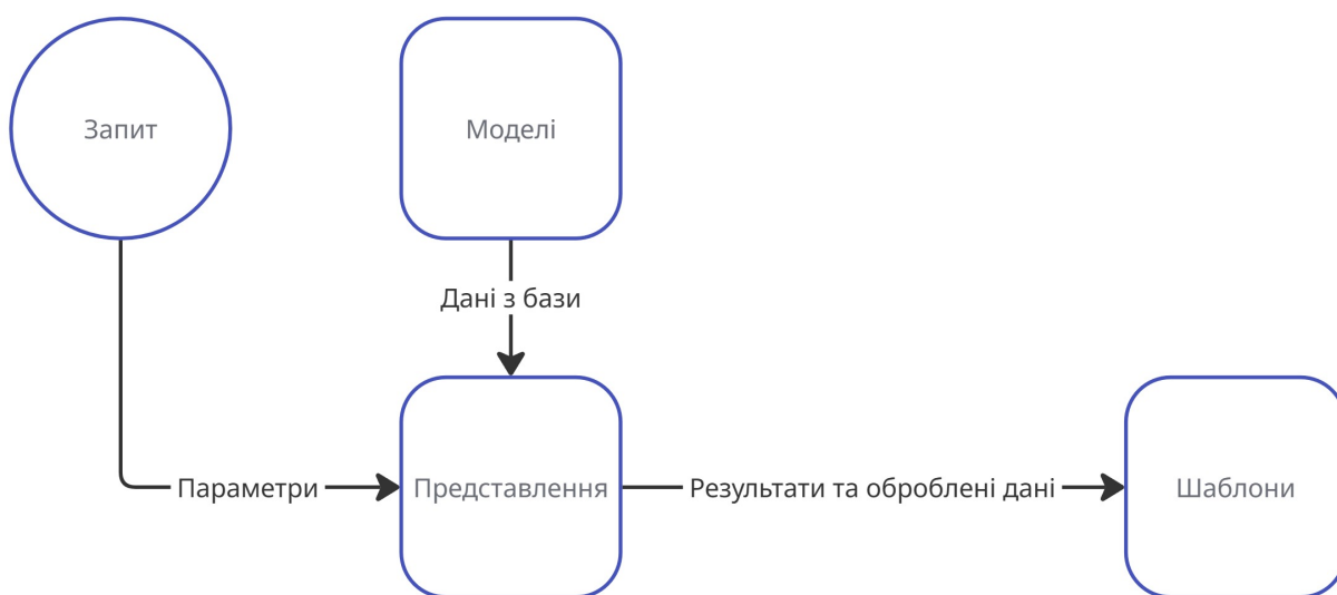
Рисунок 3. - Шаблон проєктування
